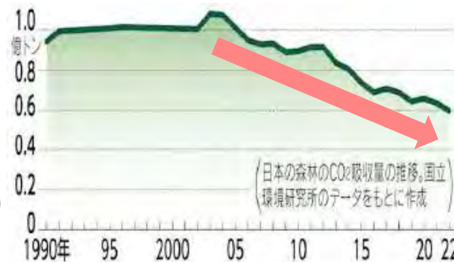
日本の森林によるCO 2 吸収量
